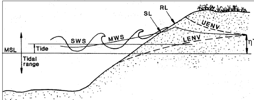
Figuur 7.1. Schematische voorstelling van de opstuwende werking van oceanische golven en getijde op de grondwaterstand in een kustaquifer (naar: Nielsen 1999).
